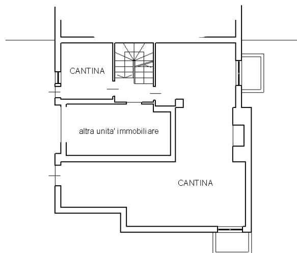
PIANO PRIMO SOTTOSTRADA (S1) H= 3.00
